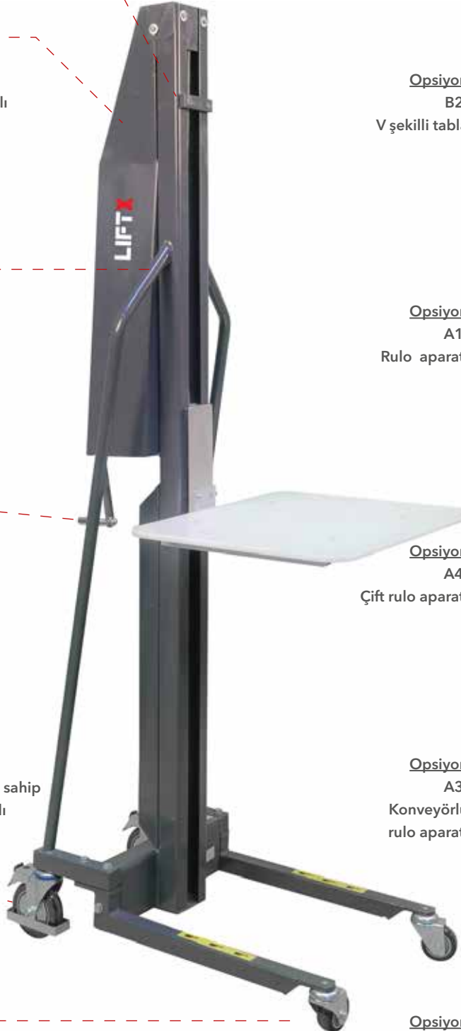
Platformu aşağı yukarı hareket etmesini sağlayan manuel el vinci
