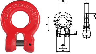
CPA Kanca Elamanı
