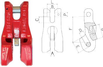
CX S Yarı Bağlantılı Kısaltma Aparatı
