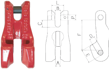
CX Kısaltma Aparatı
