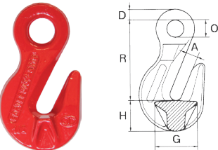
CD Kısaltma Kancası
